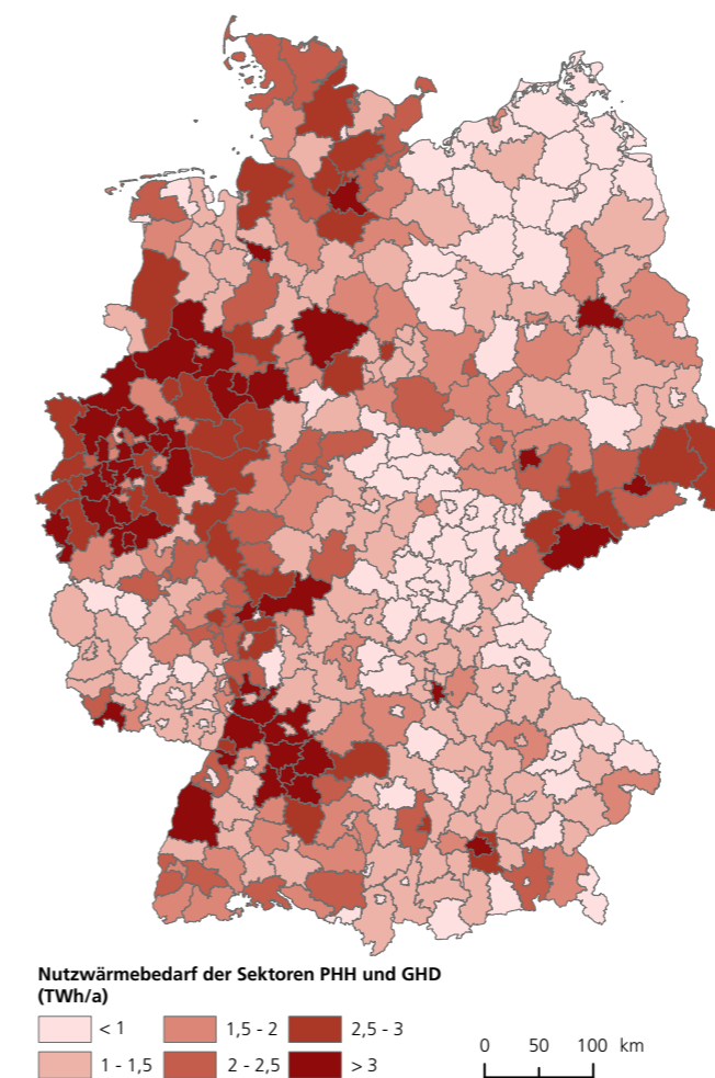
Abbildung 4: Regionale Verteilung des Nutzwärmebedarfs in Deutschland (2014) für private Haushalte (PHH) und Gewerbe, Handel, Dienstleistungen (GHD); ohne industrielle Prozesswärme (© Eikmeier, Fraunhofer IFAM) 30
