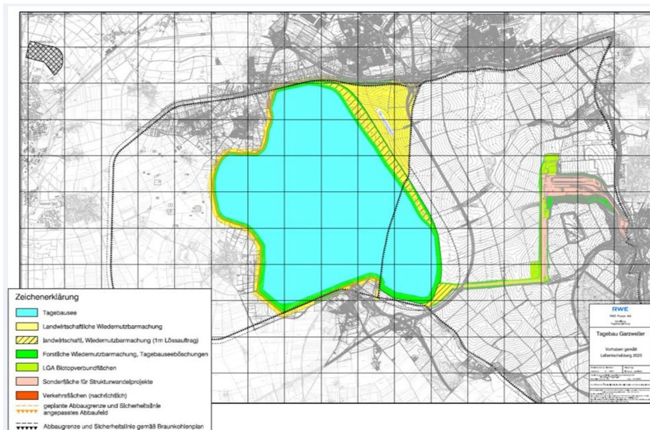
Bild 3.4 – Geplanter Tagebausee Garzweiler (Quelle: RWE Power AG)
