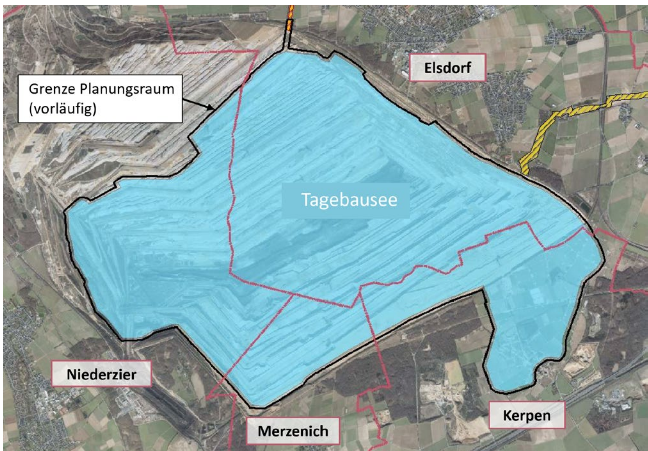
Bild 3.3 – Geplanter Tagebausee Hambach (Quelle: RWE Power AG)
