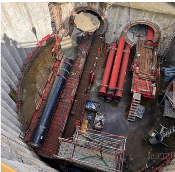
Bild 7.4 – Portale zum Düker DN 2800 und DN 3200 (Quelle: Bezirksregierung Arnsberg)
