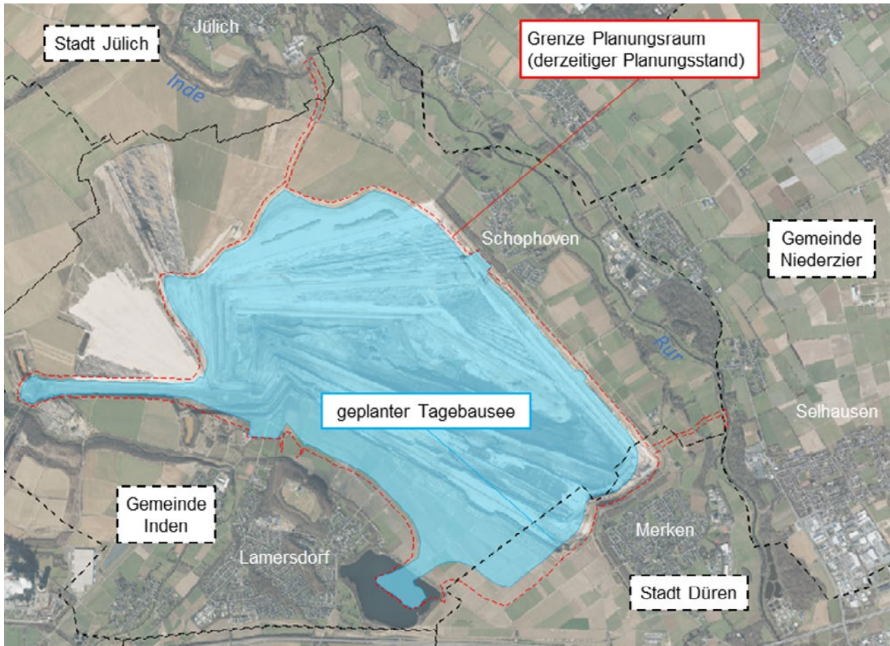
Bild 3.2 – Geplanter Tagebausee Inden (Quelle: RWE Power AG)
