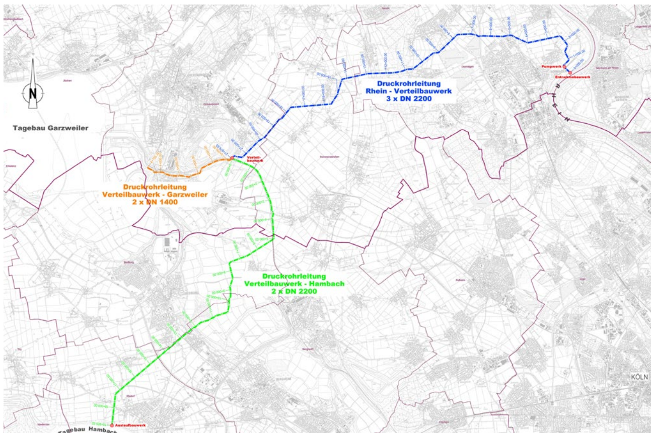
Bild 3.5 – Übersicht des Gesamtsystems der Rheinwassertransportleitung – maßstabslos (Quelle: RWE Power AG)
