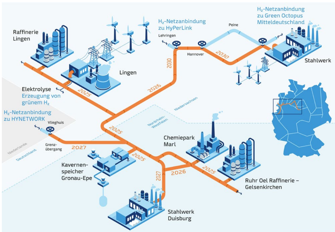
Bild 8.3 – Wertschöpfungskette Geth2 (Quelle: RWE Gas Storage West GmbH)
